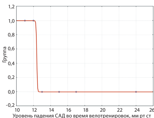
Рисунок 6. Графическое представление логит-регрессии для признака «Уровень падения САД во время велотренировок»
