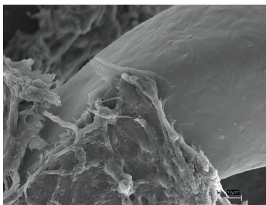
Рисунок 4. Внешняя поверхность стента, изъятото из ВОПЖ спустя 14 месяцев после имплантации
