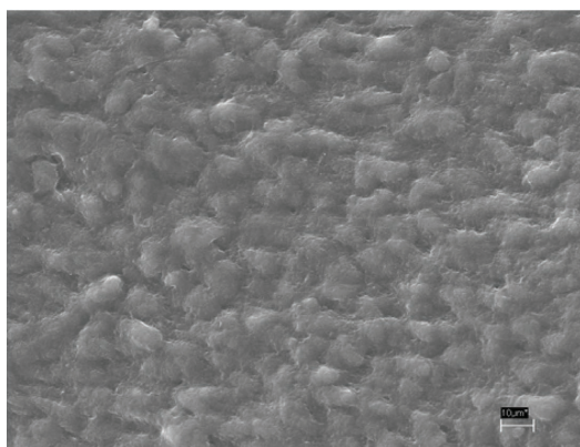
Рисунок 5. Внутренняя поверхность стента, изъятото из ВОПЖ спустя 14 мес. после имплантации
